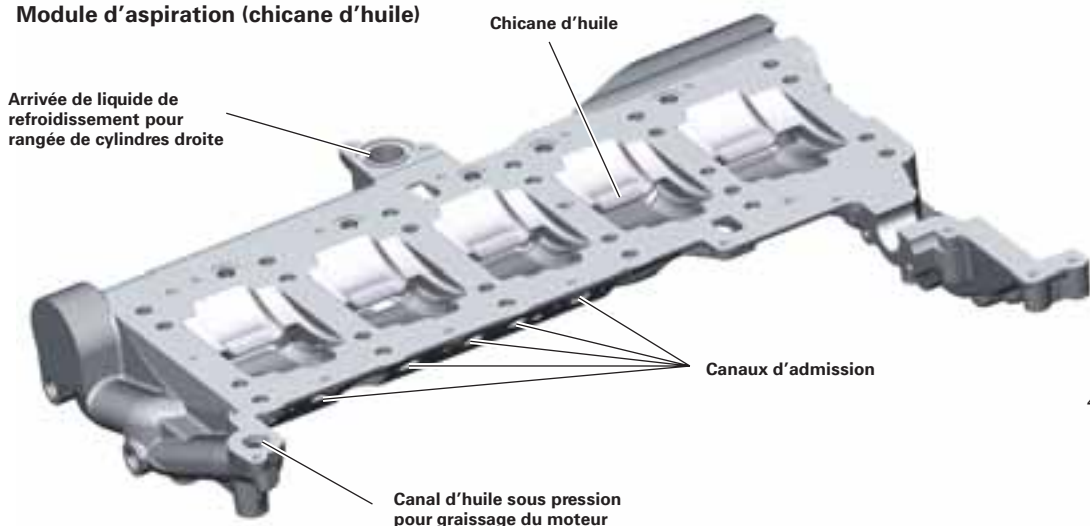
Module d'aspiration (chicane d'huile)
